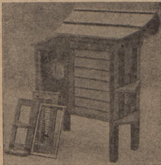
Uł Lewickiego z daszkiem podwójnym, typ pierwszy-
