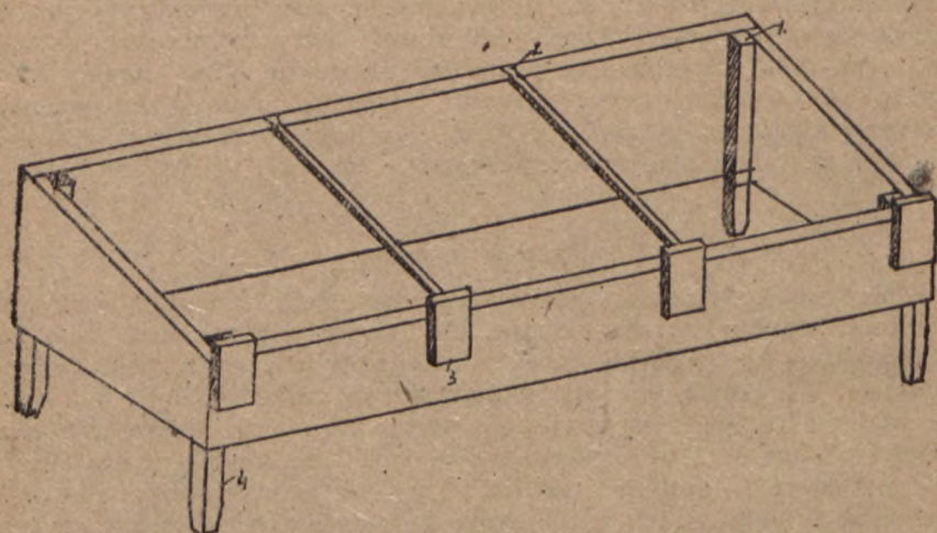
Rys. 1. Skrzynia inspektowa — 1) wiązanie skrzyni i umocnienie słupkami; 2) miecz (zaciós, złącze); 3) listwy podtrzymujące okna; 4) nogi skrzyni inspektowej.
