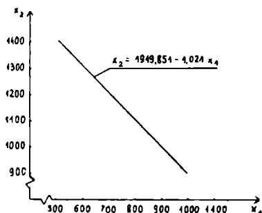
Ryc. 1. Zależność pomiędzy powierzchnią jęczmienia ( x_2 ) w tys. ha a powierzchnią owsa ( x_1 ) w tys. ha Relationship between the area of barley ( x_2 ) in thousands ha and the area of oats ( x_1 ) in thousands ha
