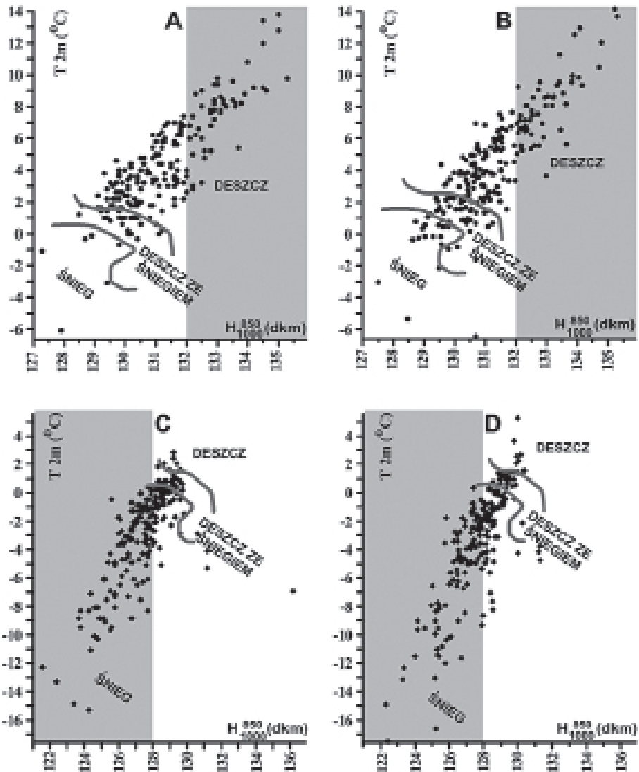
Rys. 2. Zależność pomiędzy temperaturą powietrza na 2 m n.p.g. a wysokością względną geopotencjału 850/1000 hPa w przypadku deszczu (wykresy A i B, odpowiednio dla danych z sondażu i danych z reanaliz) i w przypadku śniegu (wykresy C i D, odpowiednio dla danych z sondażu i danych z reanaliz). Szare prostokąty obejmują przypadki, podczas których stwierdzono zgodność rodzaju opadu z przyjętymi do jego określania kryteriami. Szare linie oddzielają poszczególne rodzaje opadu atmosferycznego
