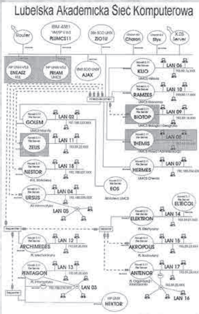
Schemat logiczny LASK z 1994 r. Zakreślone obszary oznaczają serwery planowane
